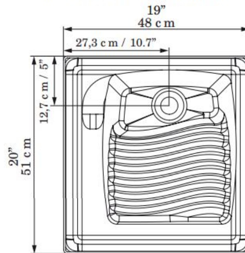
VISTA EN PLANTA / UPPER VIEW
